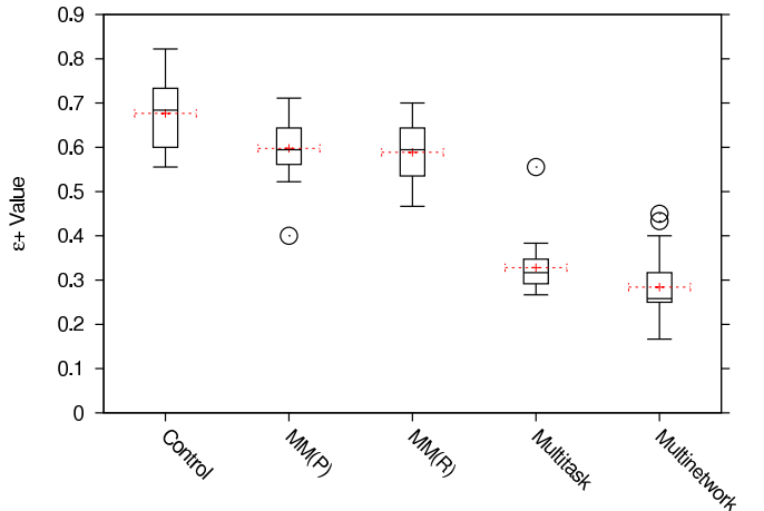
(b) I_{\epsilon+}^1 Values.
