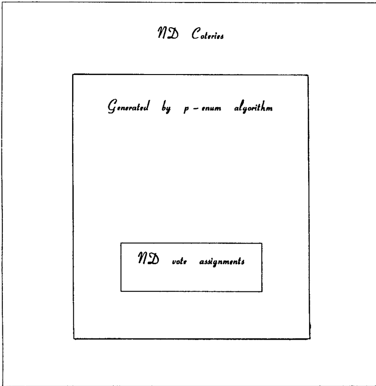
FIG. 3. Venn diagram.
