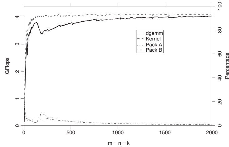
Fig. 16. Opteron (2.2 GHz).
