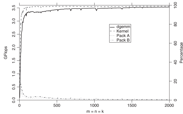
Fig. 17. Itanium2 (1.5 GHz).
